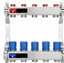
Коллекторная группа с балансировочными и термостатическими вентилями, нержавеющая сталь
